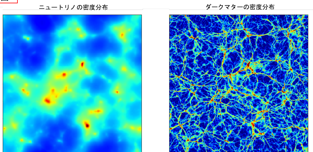
図1 宇宙大規模構造形成における、ニュートリノ（左）とダークマター（右）の密度分布。ニュートリノは質量が小さく速度分散が大きいため、広がった分布を示すのに対して、ダークマターはフィラメント構造と呼ばれるひも状の高密度領域を形成する。
