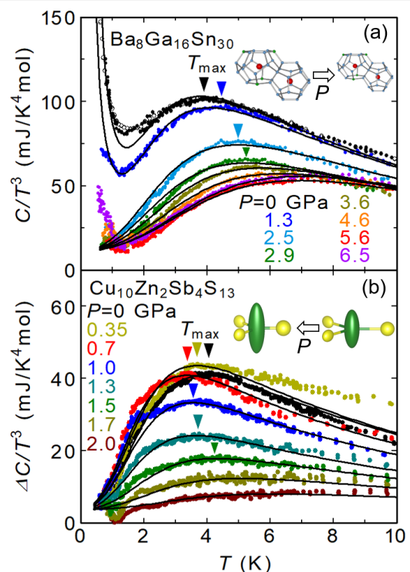
図 2. いろいろな圧力下における、(a) クラスレート \text{Ba}_8\text{Ga}_{16}\text{Sn}_{30} と (b) テトラヘドライト \text{Cu}_{10}\text{Zn}_2\text{Sb}_4\text{S}_{13} の比熱 C を温度の 3 乗で割った C/T^3 の温度変化。内挿図は加圧によるクラスレート中のカゴと、テトラヘドライトの \text{S}_3 三角形中の銅原子の振動の変化を模式的に示したもの。
