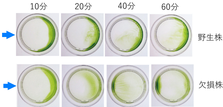
図1 暗室で行った実験の様子（上図）と、強い青色光に対するクラミドモナスの反応（下図）。シャーレ内のクラミドモナスに、矢印の方向から強い青色光を当てると、最初は、野生株、DYBLUP 欠損株ともに光源から離れるが、欠損株では順化が起き、60 分後にはほとんどが再び光源に向かう。
