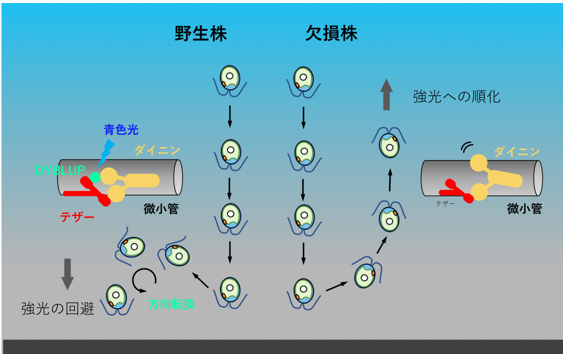
図2 DYBLUP が光順化を防止する仕組み。 光と反対の方向に移動した野生株は、一時的に光に向かう運動を示すが、すぐに方向転換して強い光を回避する。この運動調節は、DYBLUP が青色光を受容し、ダイニンとテザーの結合を安定化させることにより生じる。DYBLUP 欠損株では、ダイニンとテザーの結合が不安定で、方向転換する運動を行うことができず、強い光に順化してしまう。
