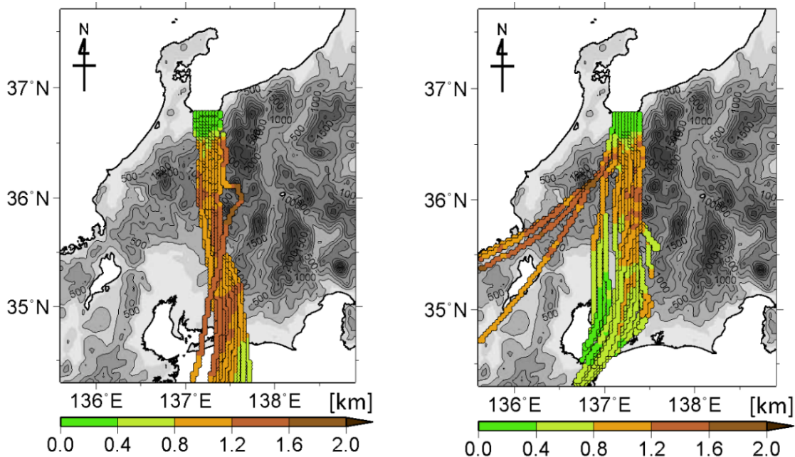
図2 数値シミュレーションと後方流跡線解析の結果。富山平野に到達した空気塊の移動経路を可視化している。左は力学メカニズムの例、右は熱力学メカニズムの例。白黒は標高。カラーは空気の移動高度。力学メカニズムの場合、濃尾平野と飛騨高地の上空を移動し山を越えて降りてきていることが分かる。一方、熱力学メカニズムの場合、濃尾平野上の低い高度から飛騨高地を乗り越えて降りてきていることが分かる。
