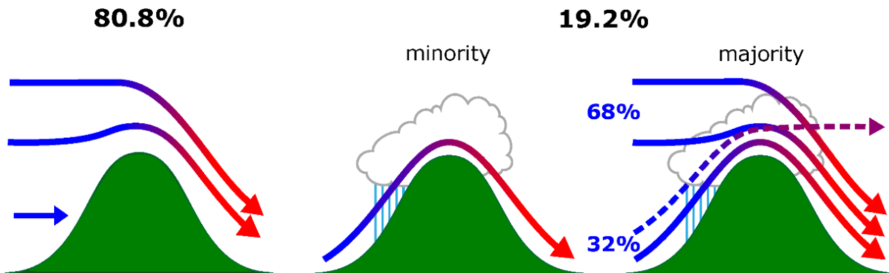
図1 フェーン現象のメカニズムと発生割合。
