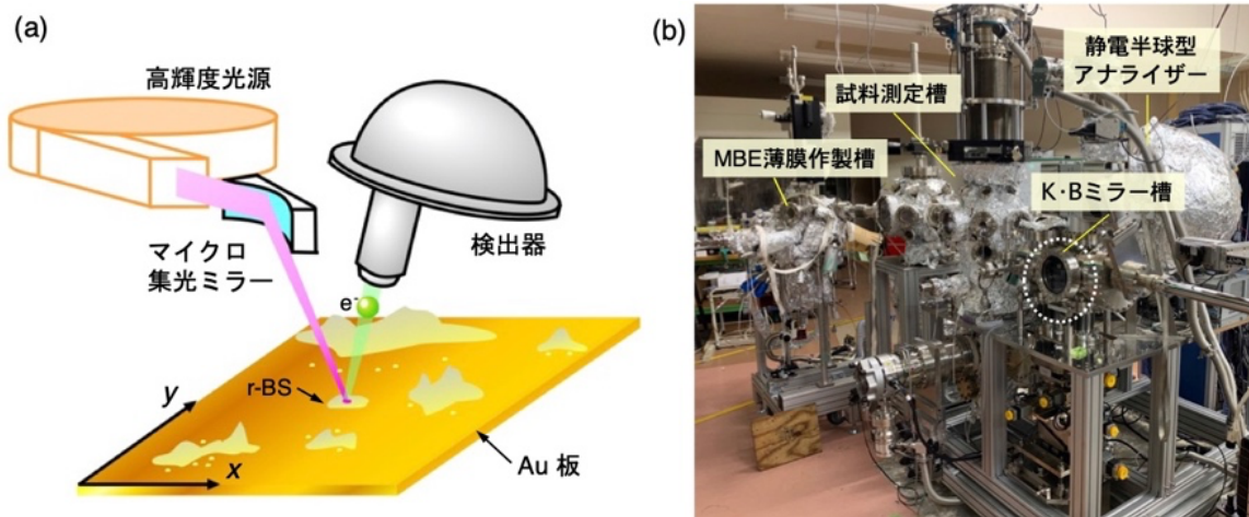
図 2: マイクロ ARPES の(a)概念図と(b)マイクロ ARPES 装置の写真。高輝度紫外線を物質表面に照射して外部光電効果によって放出された光電子のエネルギーと運動量を精密に測定することで、物質の電子構造を決定できます。さらに光のスポットサイズをミクロン単位まで小さくすることで、原子層物質などにおける局所電子構造の決定が可能になります。本研究では、Au 基板上に拡散した r-BS 試料にピンポイントでマイクロ紫外線を照射することで、r-BS の電子状態を精密に明らかにしました。
