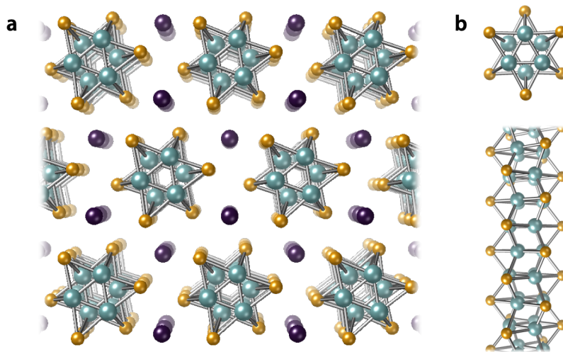
図1 (a) 三元系TMCの結晶、(b) 単一のTMC原子細線の模式図。緑色が遷移金属原子、橙色がカルコゲン原子、紫色が挿入原子に対応する。
