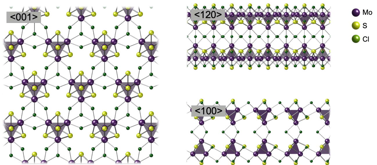
図2 超原子層「 \text{Mo}_8\text{S}_8\text{Cl}_{11} 」のモデル図。 \langle 001 \rangle 、 \langle 120 \rangle 、 \langle 100 \rangle はそれぞれ、異なる方向から \text{Mo}_8\text{S}_8\text{Cl}_{11} を見た際の配列を示す。
