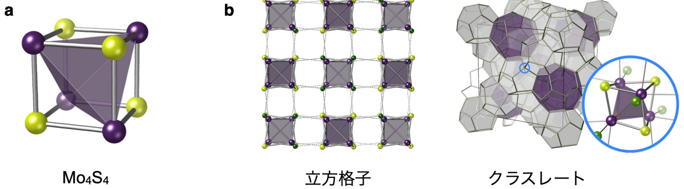
図1 (a) 立方体型の超原子 \text{Mo}_4\text{S}_4 クラスターと (b) 先行研究で報告されていた三次元集積体のモデル図。
