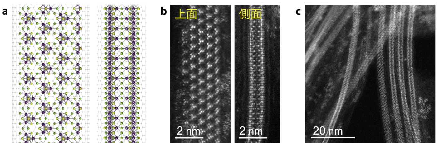
図3 (a) カーボンナノチューブの内部空間に成長した \text{Mo}_8\text{S}_8\text{Cl}_{11} ナノリボンのモデル図および (b, c) 透過電子顕微鏡写真。モデル図と同様の構造が安定して存在している。
